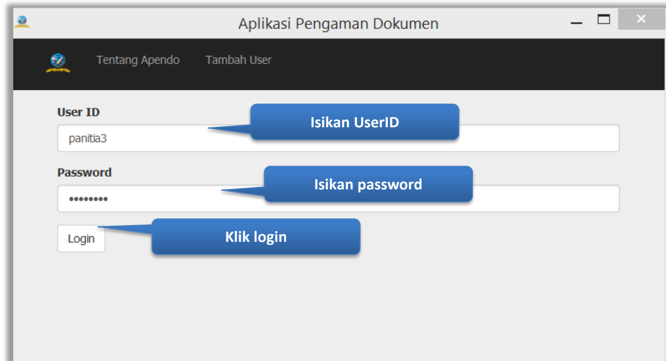
Gambar 8. Halaman Login
