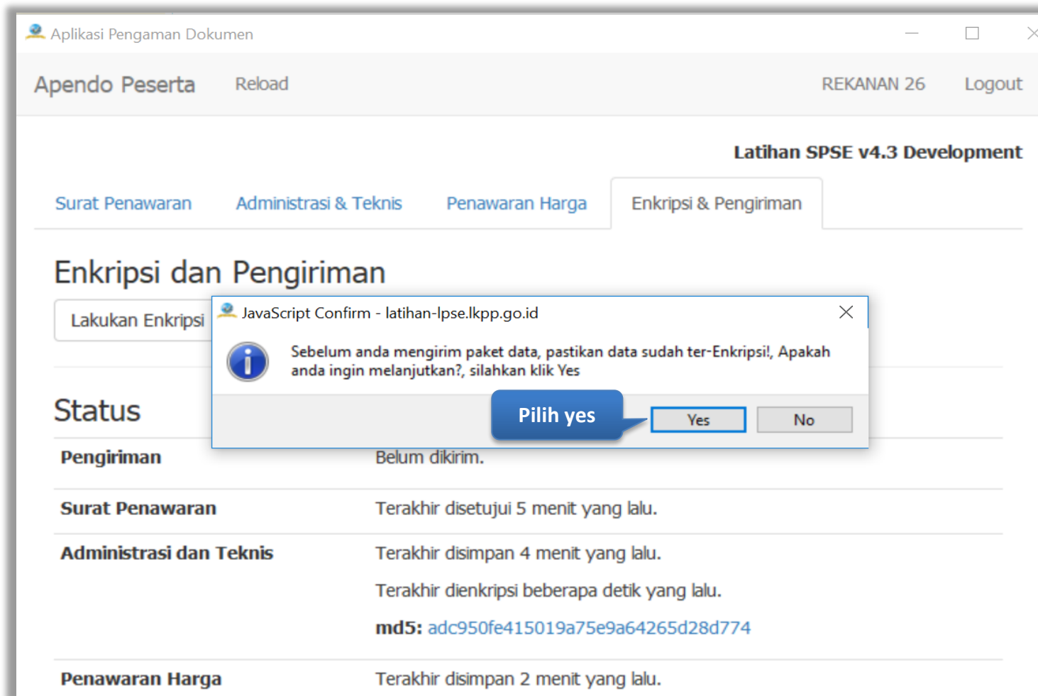
Gambar 25. Konfirmasi Apendo
