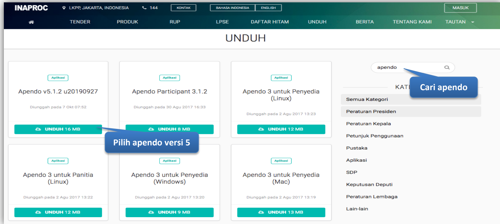
Gambar 1. Halaman Inaproc
