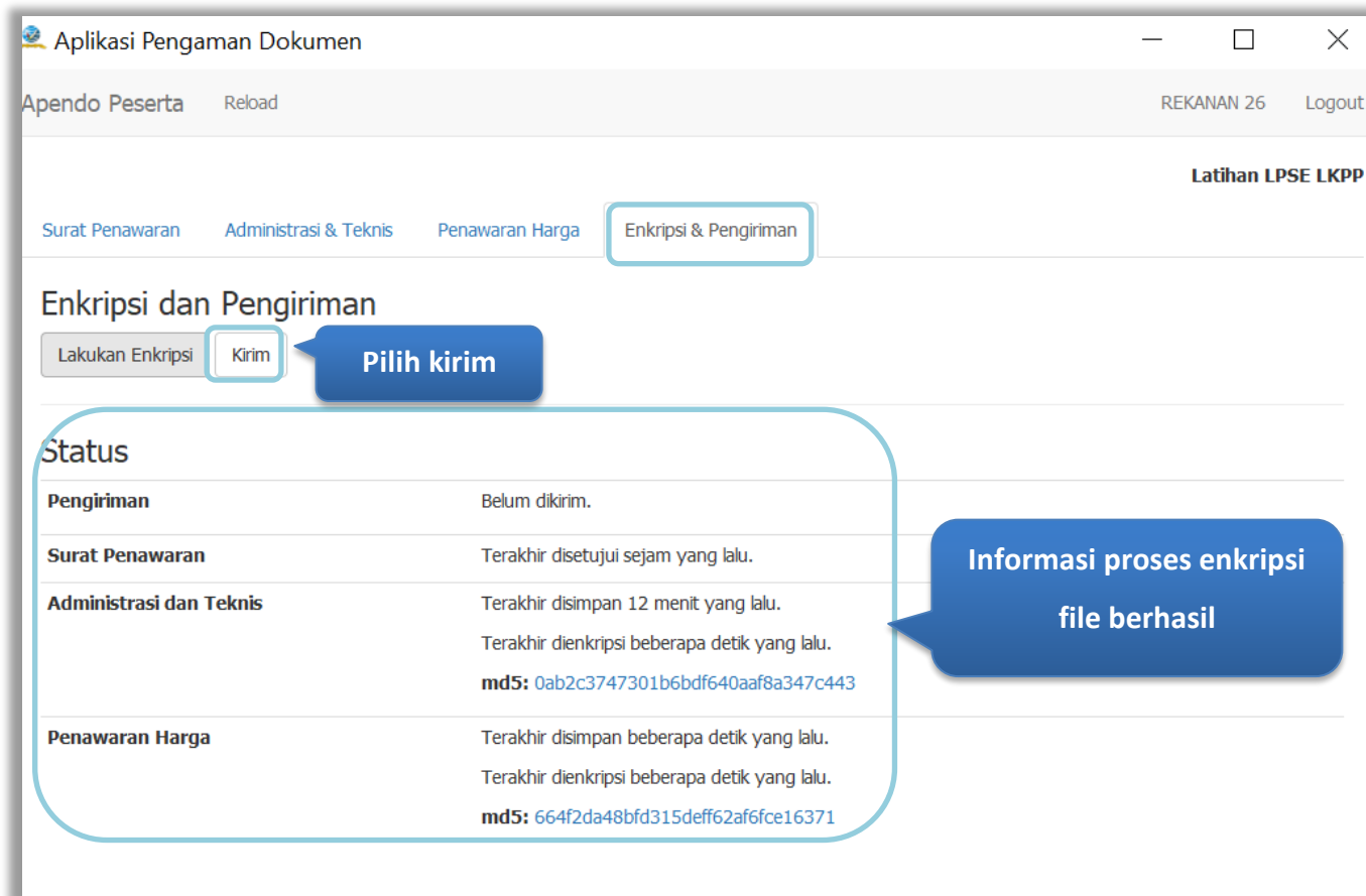
Gambar 24. Kirim Penawaran
